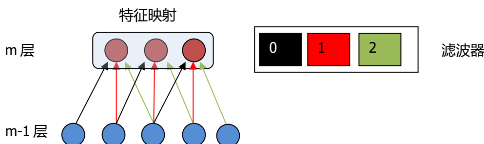
图 5.4: 特征映射
