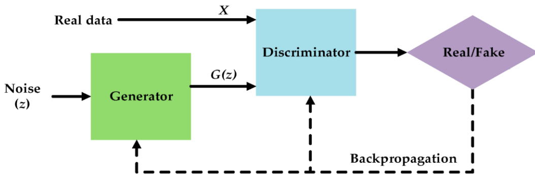
图 14.3 GAN 的结构
