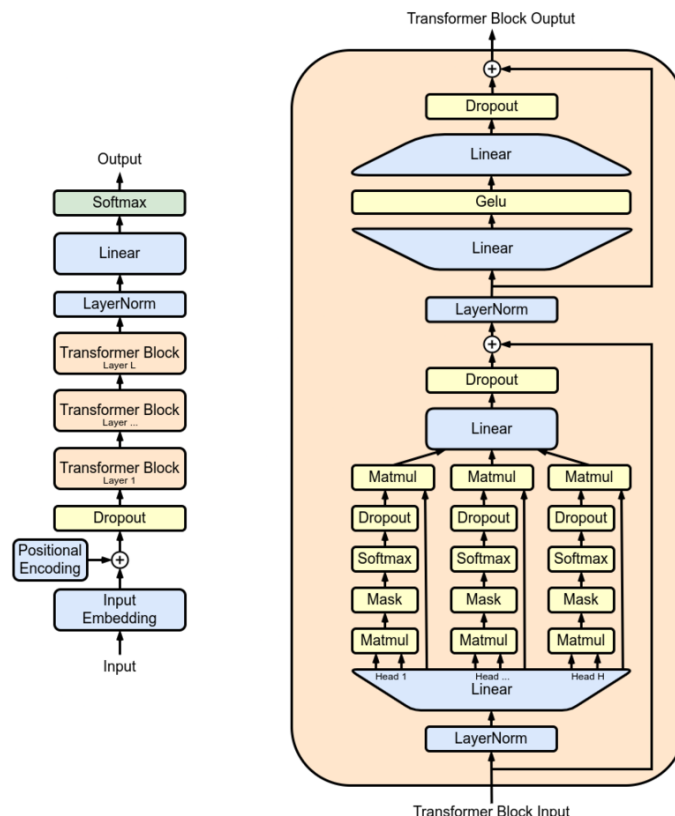
图 12.11 GPT 的结构
