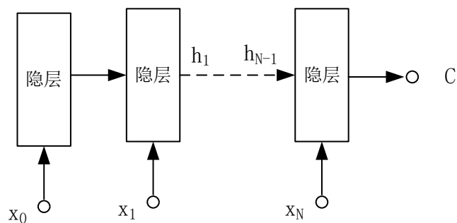
图 10.2 Encoder 结构
