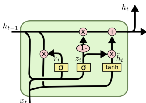
图 8.24 GRU
