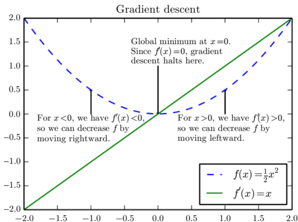
图 2.10 梯度下降
