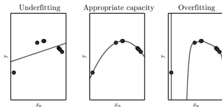
图 14.4 模型拟合
