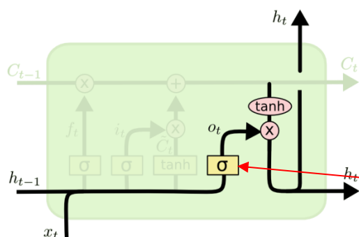
图 8.21 LSTM 块的第四层
