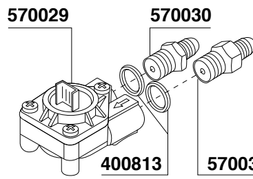
570029
