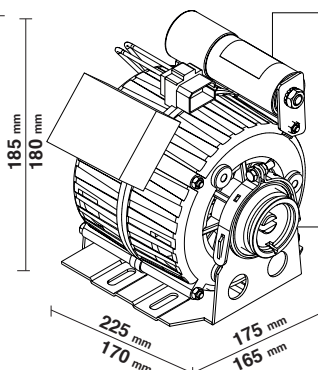
621113 =25µF
