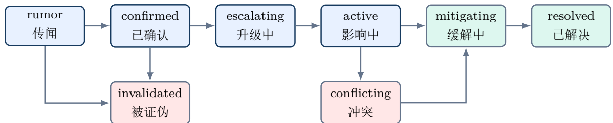
图 18: 风险事件时序状态机
