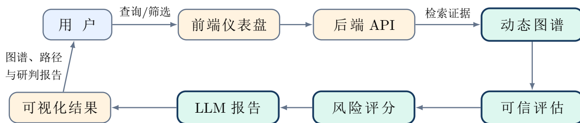
图 11: 系统交互闭环流程
