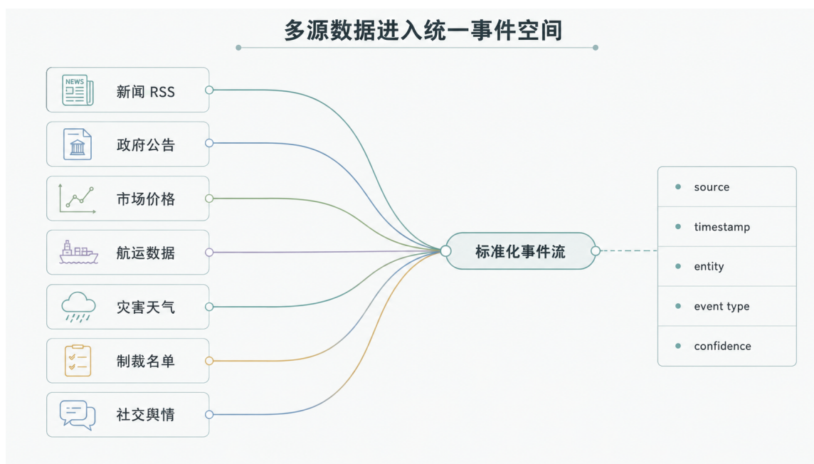
图 15: 多源数据接入架构
