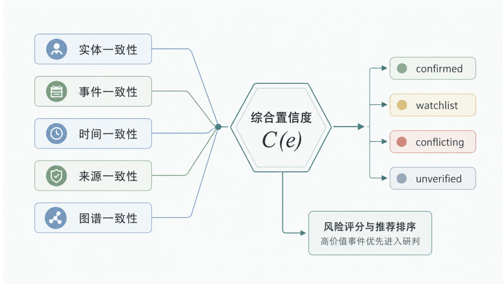
图 6: 多层一致性驱动的可信融合机制
