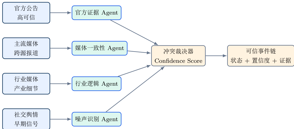
图 19: Trust Graph 驱动的多 Agent 冲突消解机制
