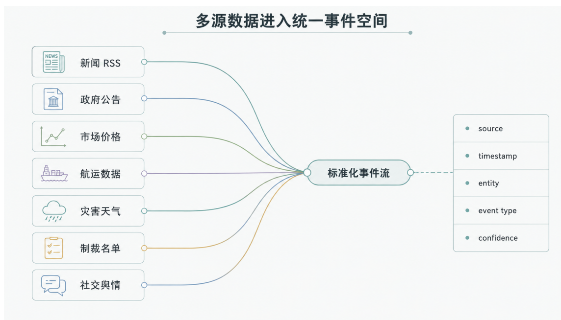
图 14: 多源数据接入架构
