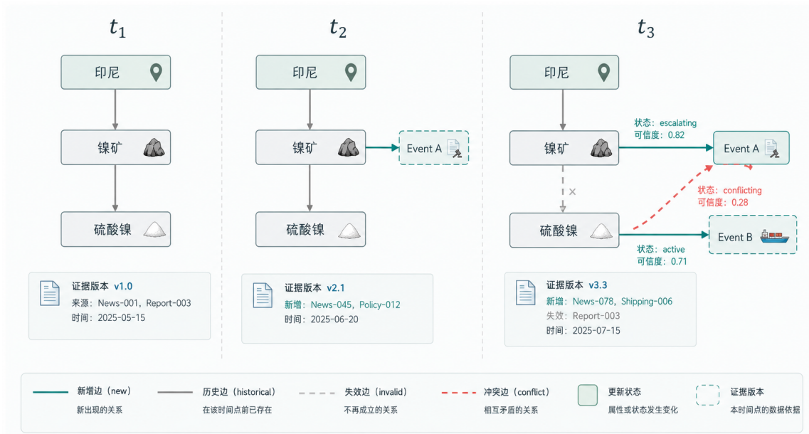
图 16: 时序可信动态图谱构建流程
