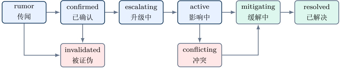
图 17: 风险事件时序状态机
