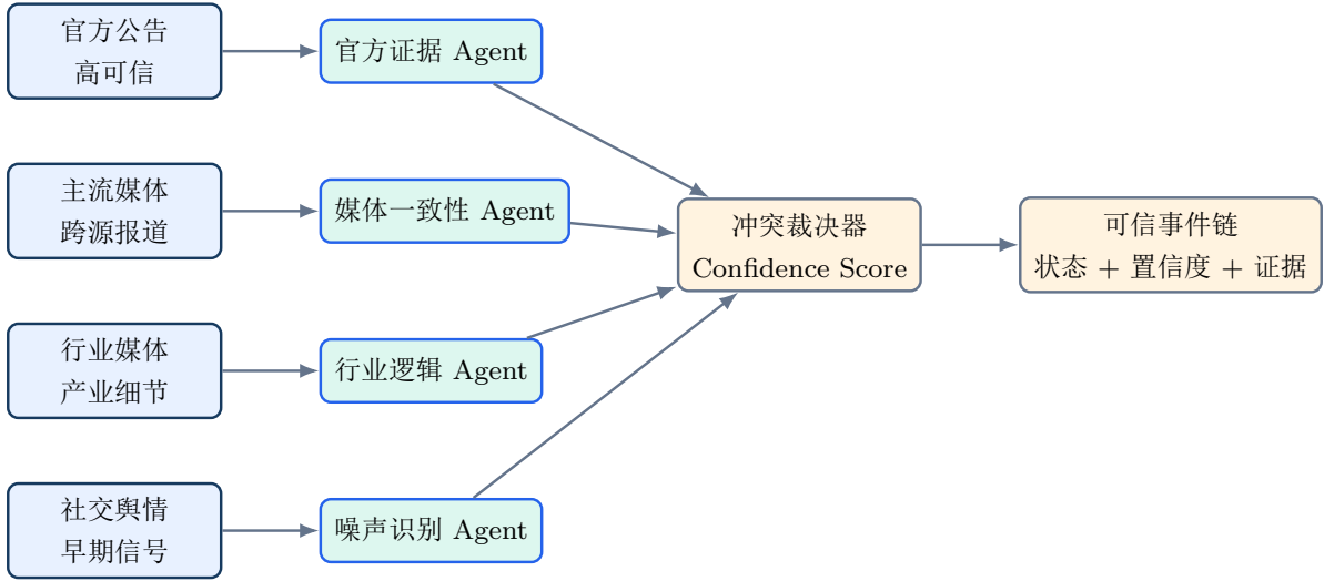
图 18: Trust Graph 驱动的多 Agent 冲突消解机制
