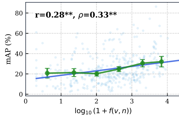
(g) T→V mAP
