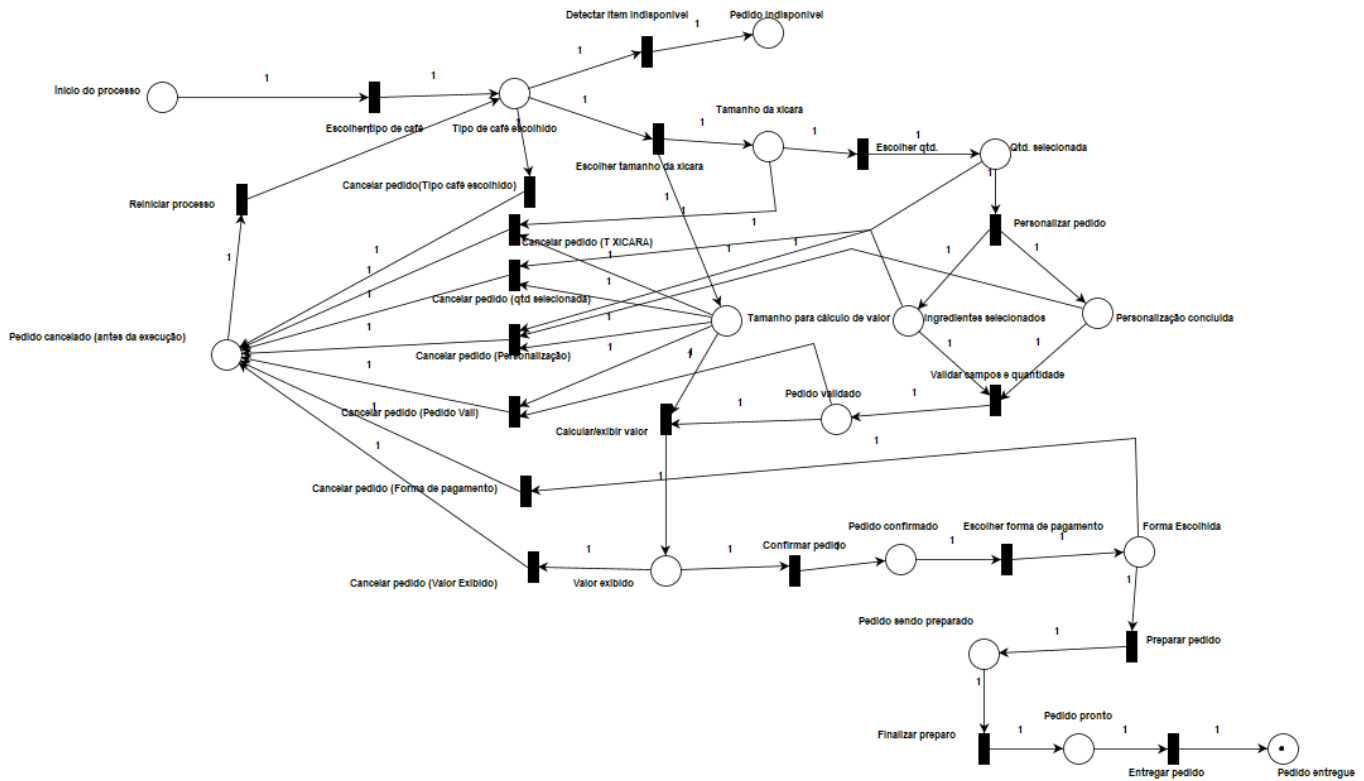
Figura 1. Rede de Petri para o sistema de máquina de café.
