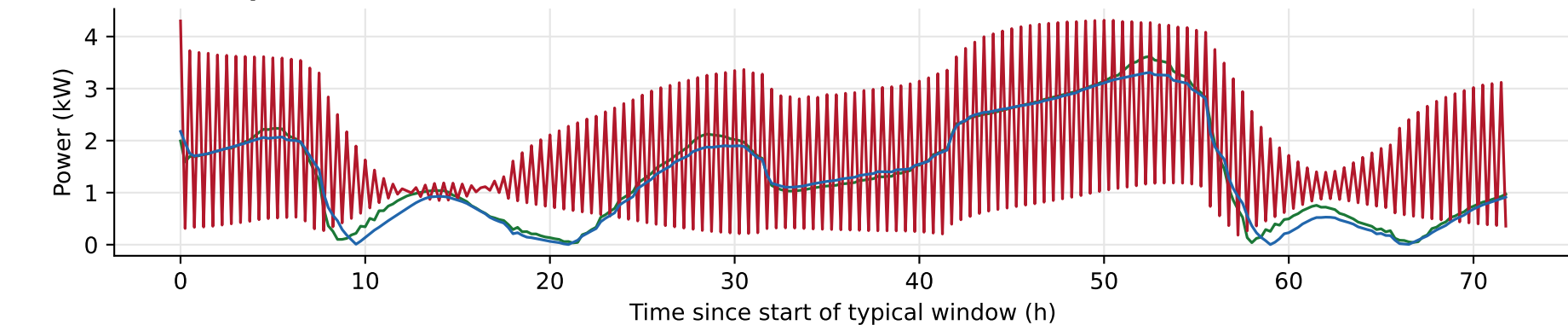
(d) HVAC power
