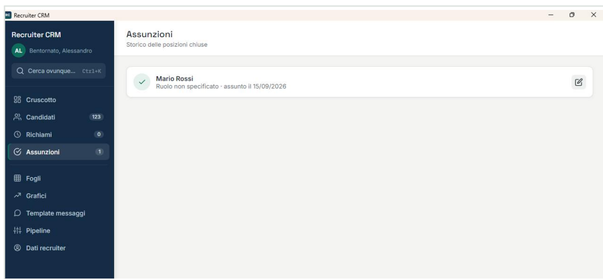
sezione Assunzioni
