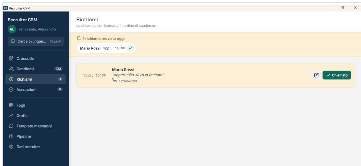
sezione Richiami
