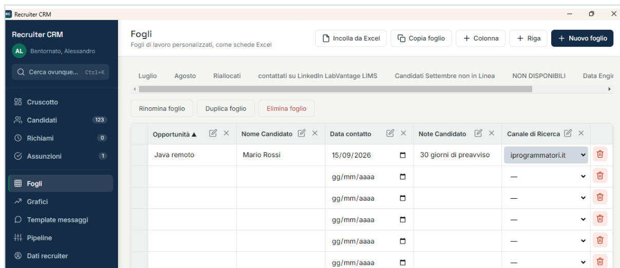
sezione Fogli
