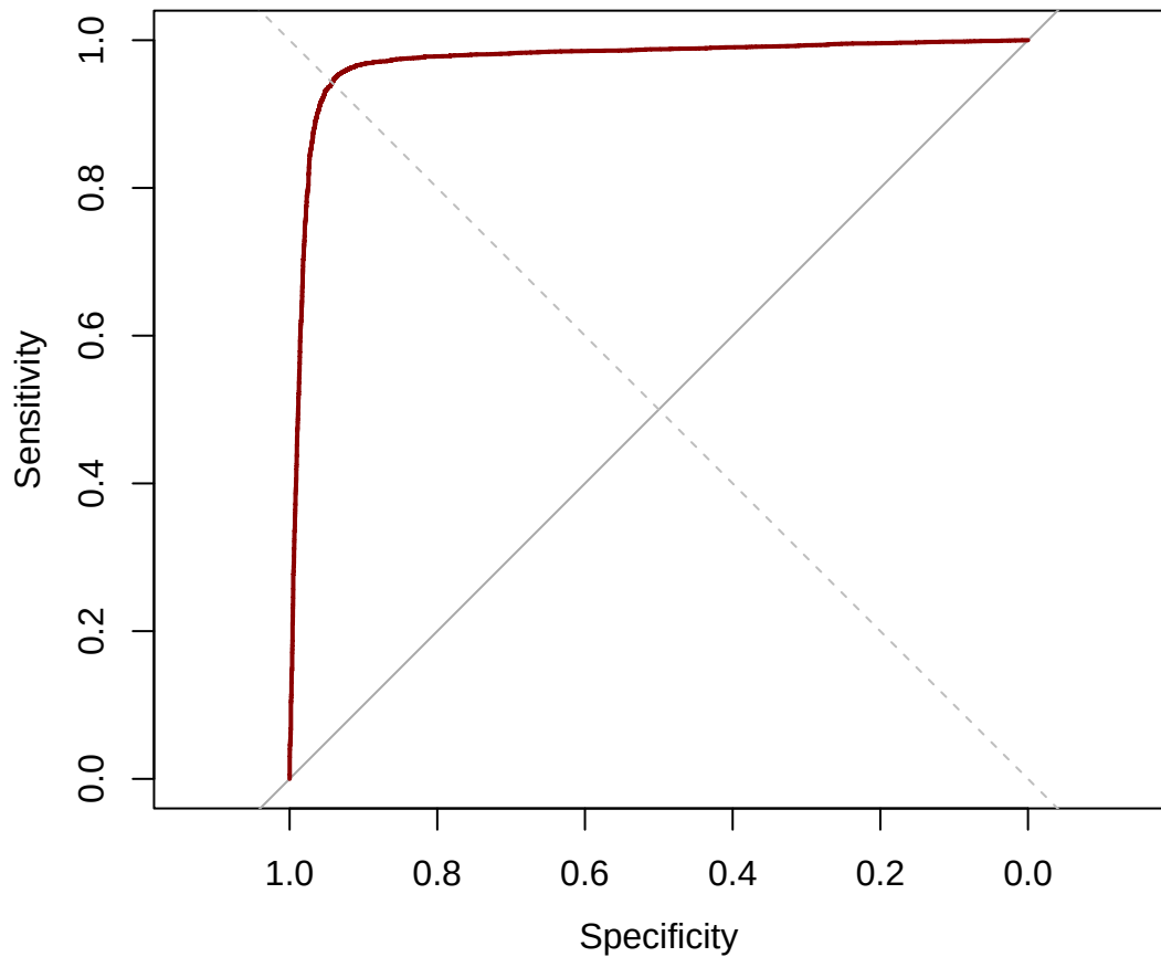
Random Forest ROC (AUC=0.9719)
