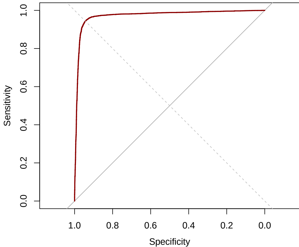
Random Forest ROC (AUC=0.9721)
