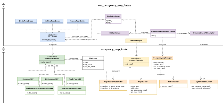
Рисунок 5 — Диаграмма компонентов программного комплекса Окупанси Мап Fusion на языке UML.
