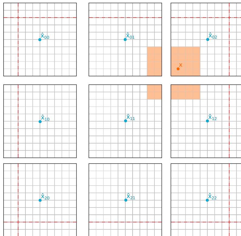
Рисунок 4.12 — Двумерная реализация локальной карты проходимости пространства с полным обновлением без блокировок.
