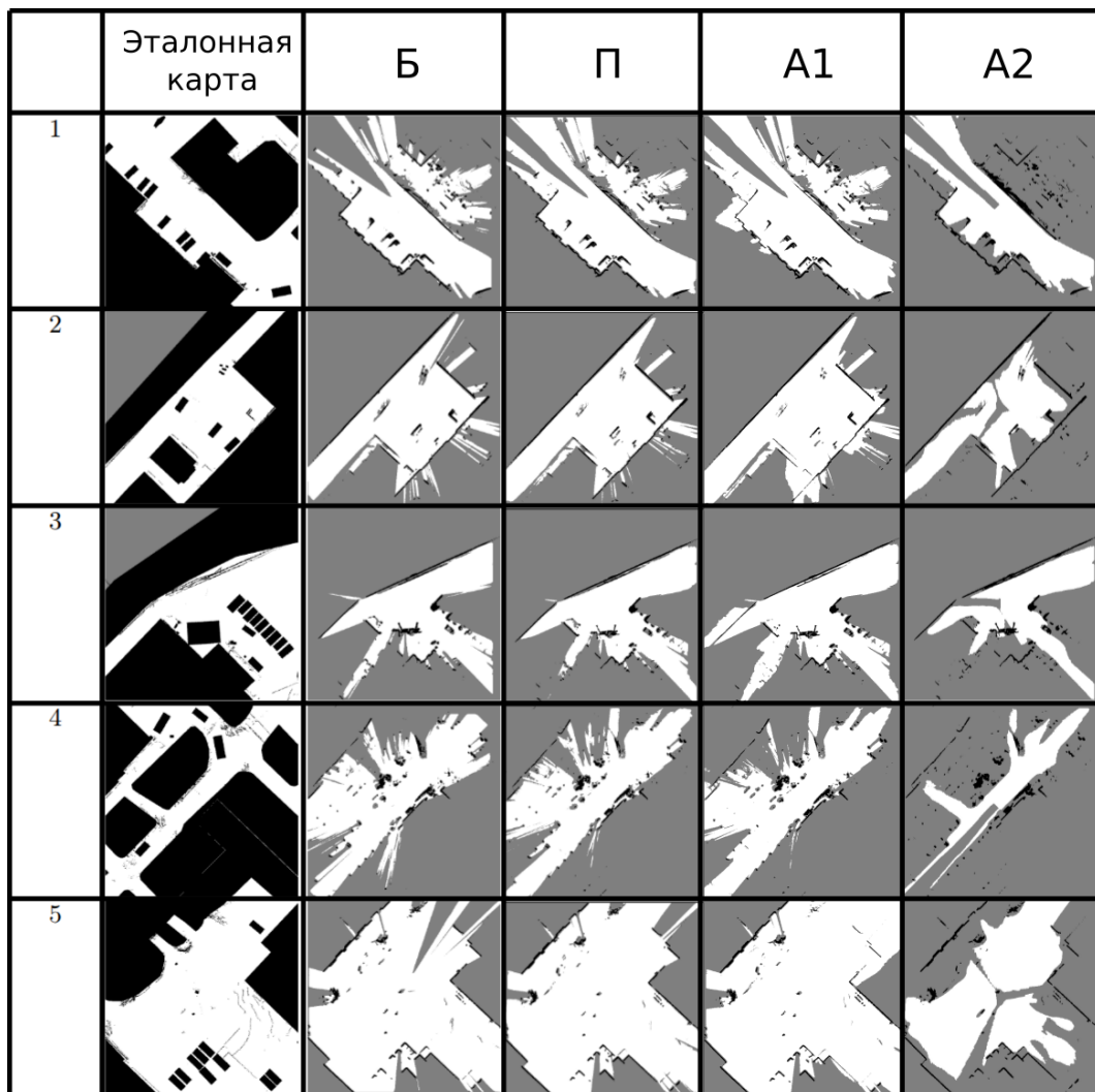
Рисунок 2.22 — Карты проходимости пространства, построенные сравниваемыми алгоритмами на тестовых данных.
