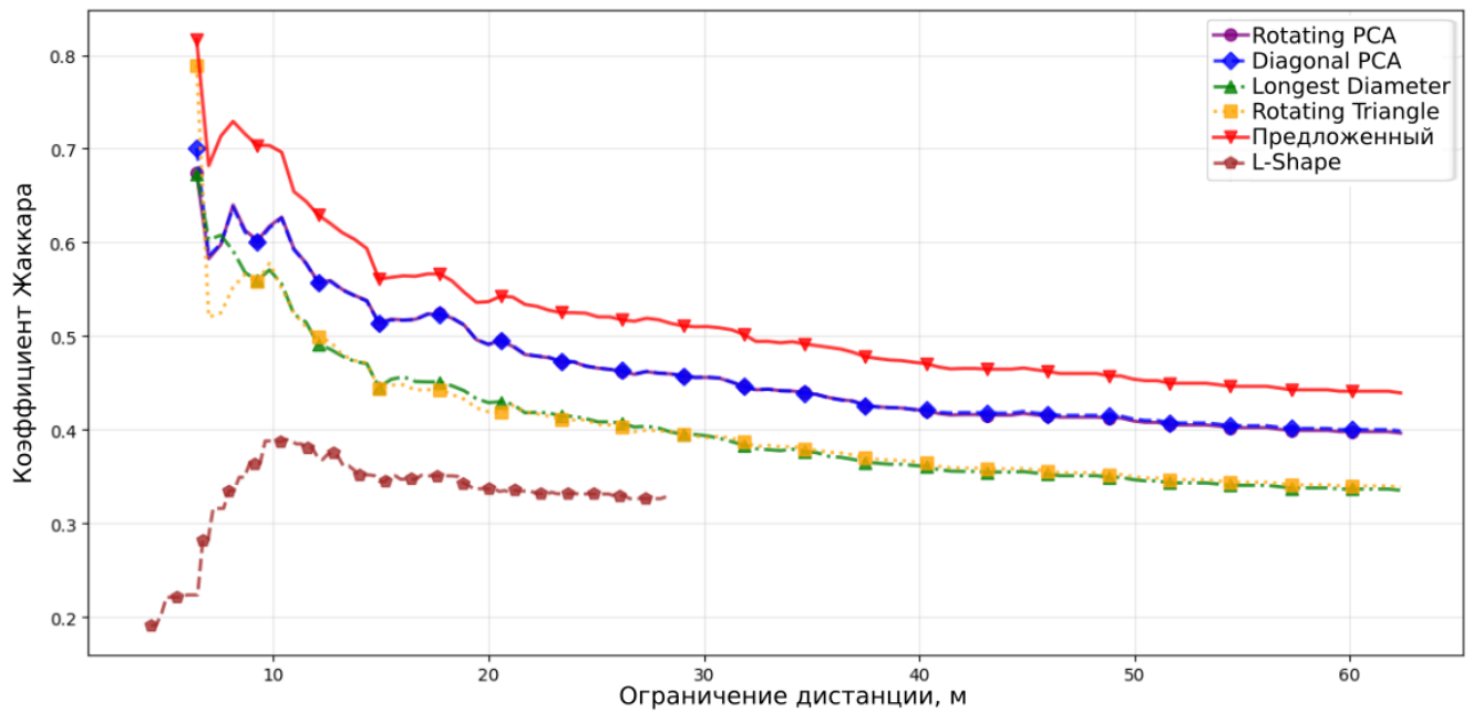
Рисунок 2.12 — График зависимости среднего коэффициента Жаккара от ограничения дистанции до детектируемых препятствий для алгоритма комплексирования и алгоритмов, не использующих комплексирование.
