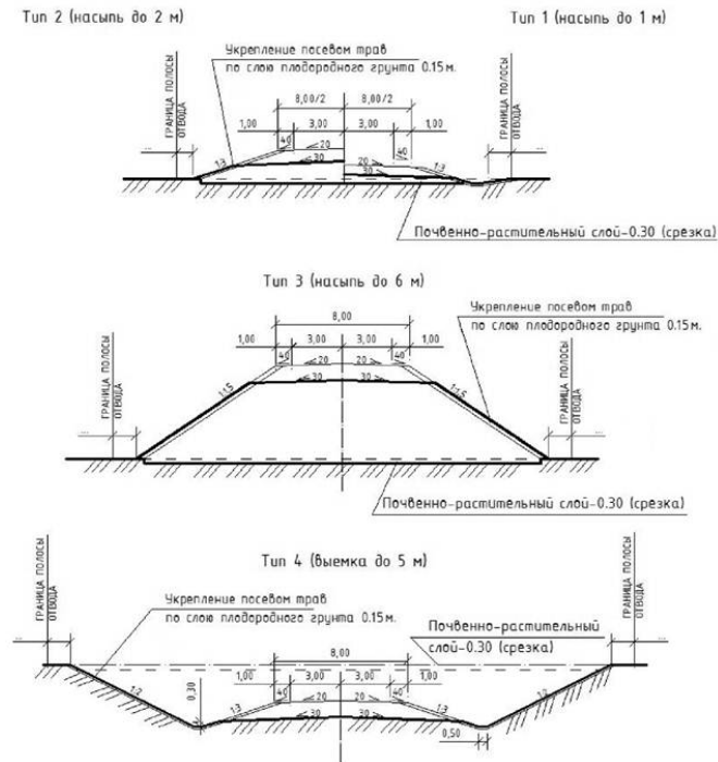
Рисунок 2.8 — Примеры оформления поперечного профиля из ГОСТ 21.701-2013 [108].
