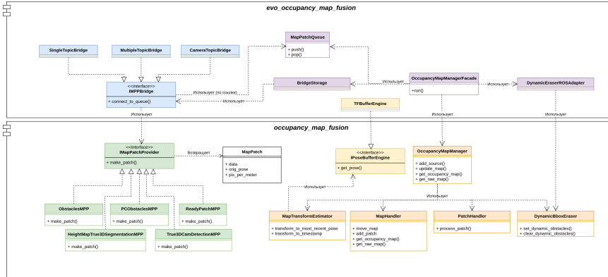
Рисунок 5 — Диаграмма компонентов программного комплекса Occupancy Map Fusion на языке UML.
