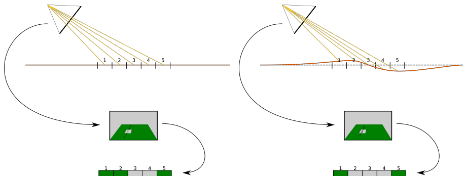
Рисунок 3 — Проецирование сегментации проезжей части на плоскость z_l = 0 (слева) и на оценённую поверхность z = z(x, y) (справа). Для облегчения восприятия проецируемая сетка представлена одним рядом.
