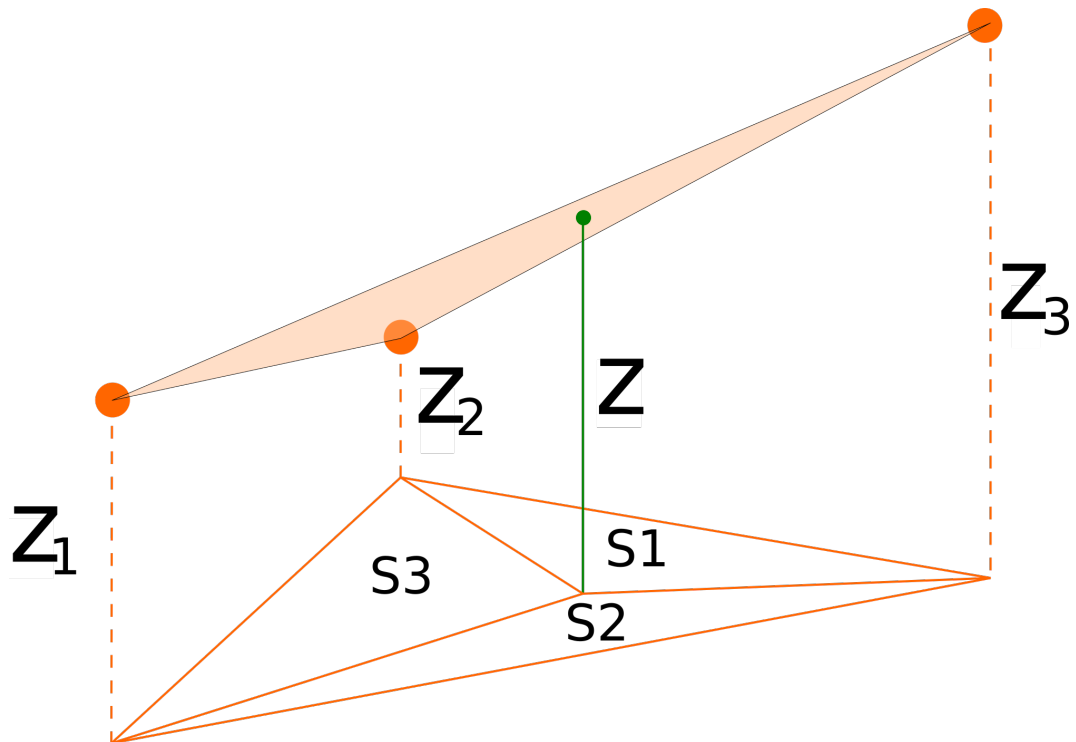
Рисунок 2.15 — Линейная интерполяция z в треугольнике.
