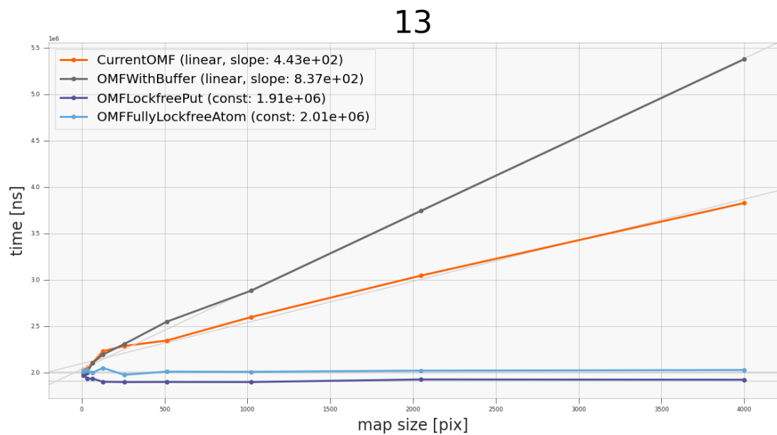
Рисунок 4.13 — График зависимости времени добавления фрагмента на карту в 13 потоках от размера карты.
