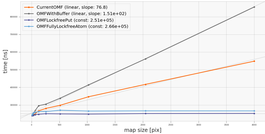
Рисунок 4.11 — График зависимости времени добавления фрагмента на карту в 5 потоках от размера карты.
