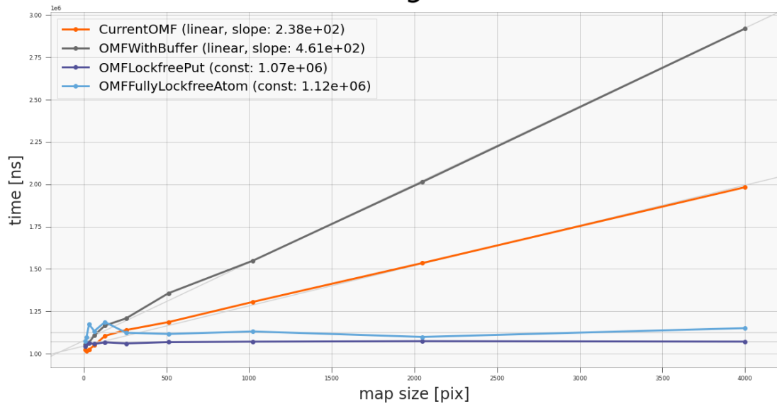
Рисунок 4.12 — График зависимости времени добавления фрагмента на карту в 9 потоках от размера карты.
