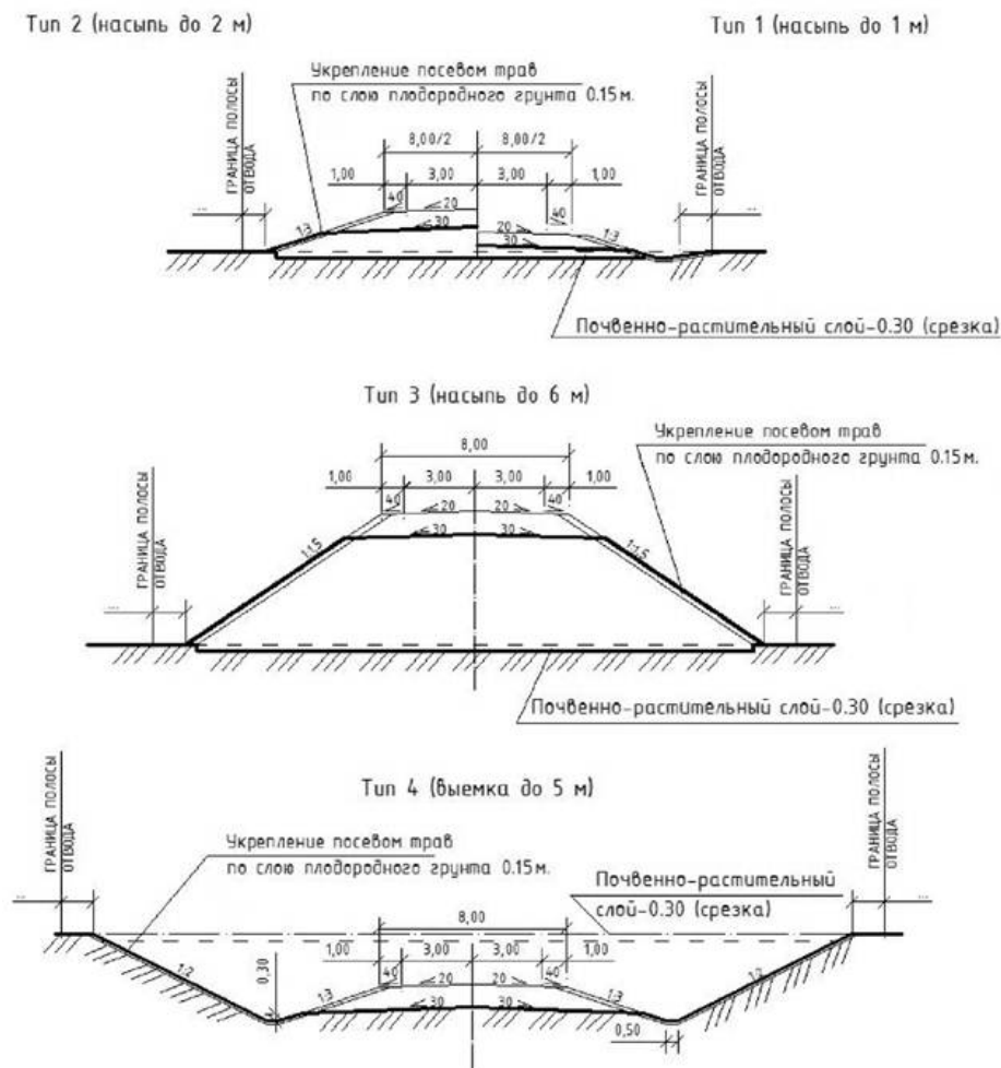
Рисунок 2.8 — Примеры оформления поперечного профиля из ГОСТ 21.701-2013 [78].
