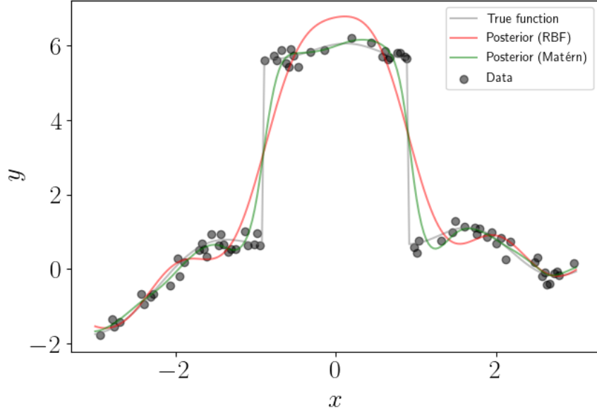
Рисунок 2.10 — Сравнение регрессии на основе гауссовских процессов с использованием в качестве ядра радиальной базисной функции и ядра Матерна [84].
