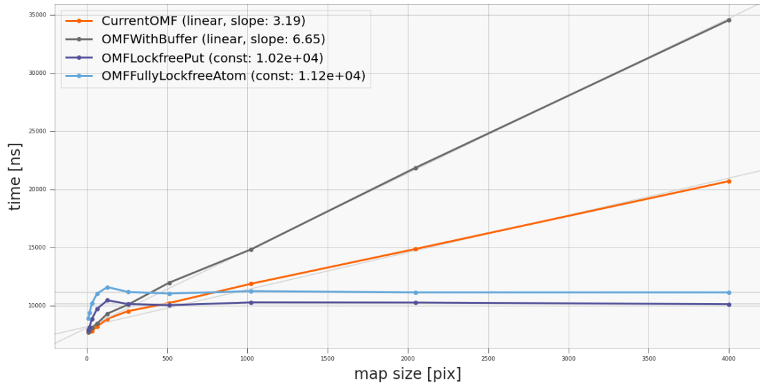
Рисунок 4.9 — График зависимости времени добавления фрагмента на карту в 1 потоке от размера карты.
