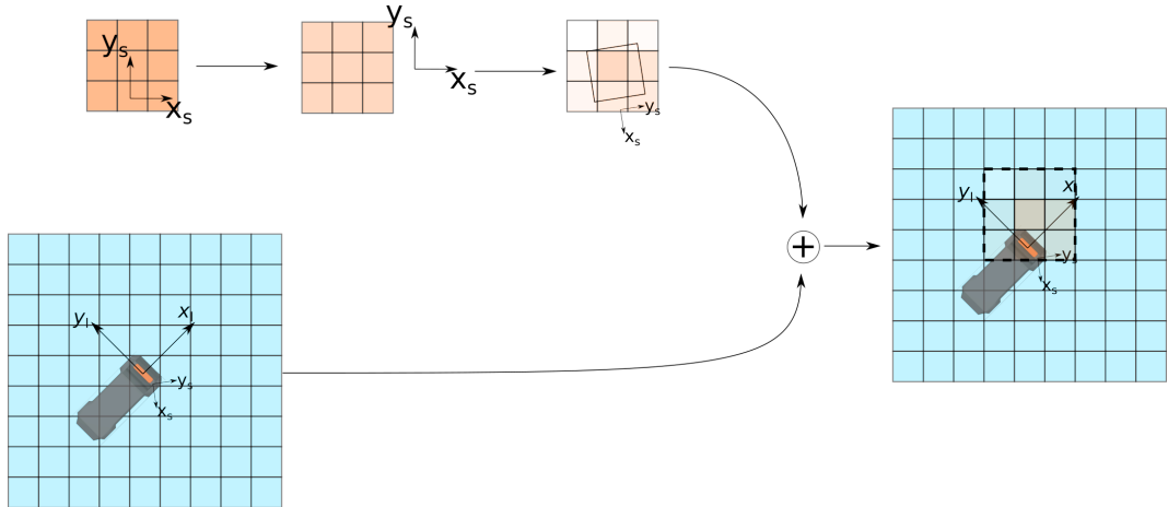
Рисунок 4.3 — Иллюстрация алгоритма добавления фрагмента от источника данных s на локальную карту проходимости пространства.
