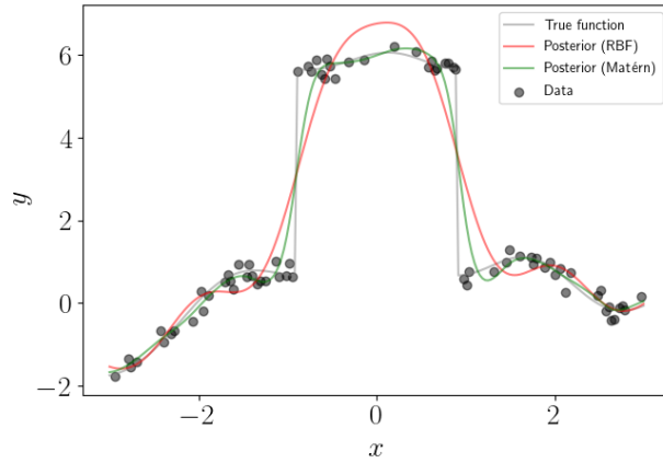
Рисунок 2.10 — Сравнение регрессии на основе гауссовских процессов с использованием в качестве ядра радиальной базисной функции и ядра Матерна [106].
