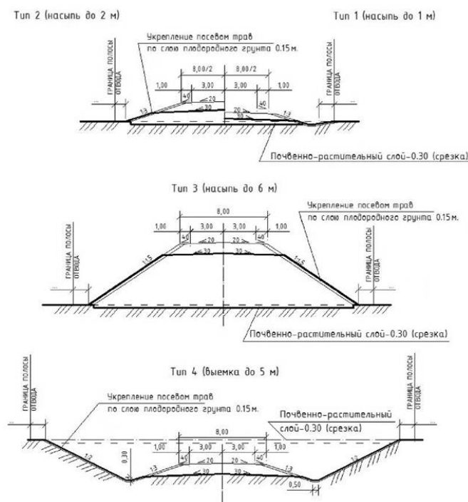
Рисунок 2.8 — Примеры оформления поперечного профиля из ГОСТ 21.701-2013 [102].
