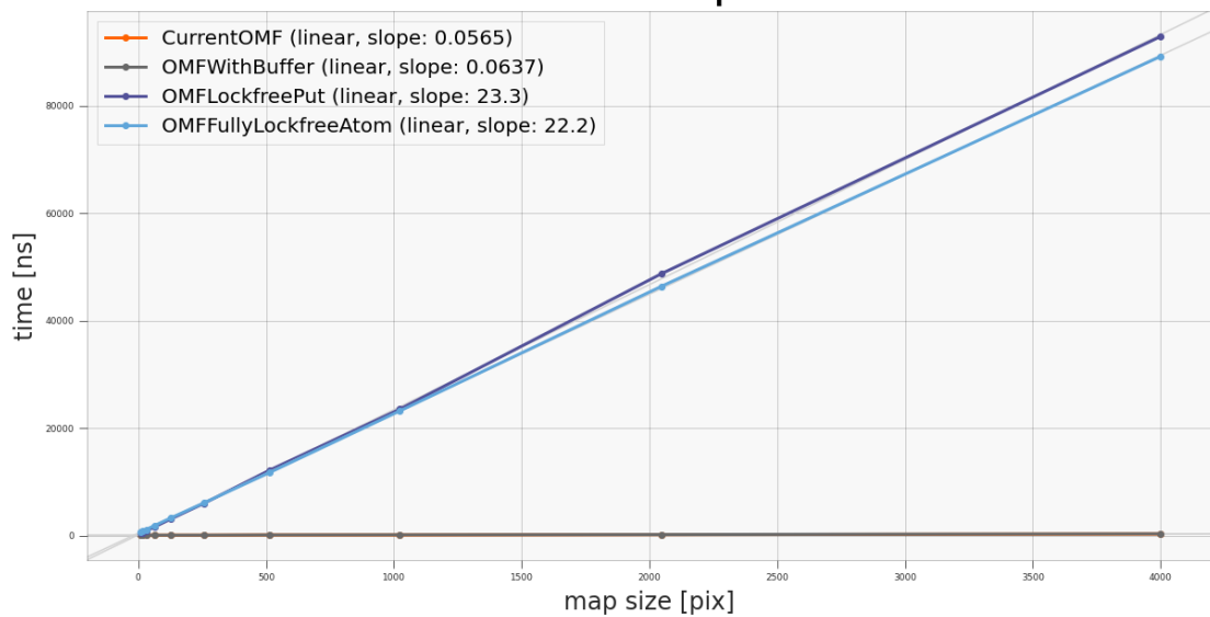
Рисунок 4.13 — График зависимости времени получения карты от её размера. График BaseOGM практически полностью совпадает с OMFWithBuffer и на таком масштабе они не отличимы.
