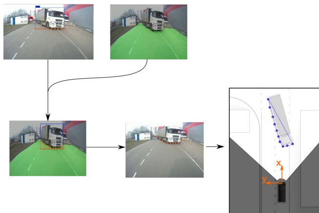
Рисунок 1 — Проекция двумерной ограничивающей рамки на вид сверху с учётом сегментации проезжей части.
