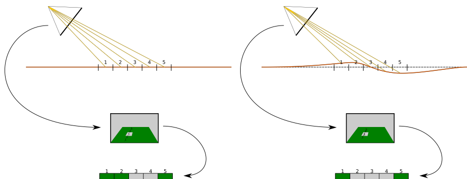
Рисунок 3 — Проецирование сегментации проезжей части на плоскость z_l = 0 (слева) и на оценённую поверхность z = z(x, y) (справа).
