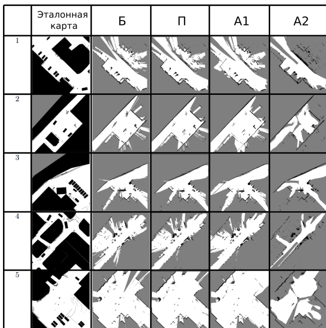
Рисунок 4 — Эталонные карты проходимости пространства и карты, построенные сравниваемыми алгоритмами на тестовых данных.
