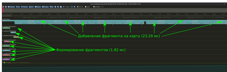
Рисунок 6 — Задержки обновления карты проходимости пространства при восьми источниках данных.
