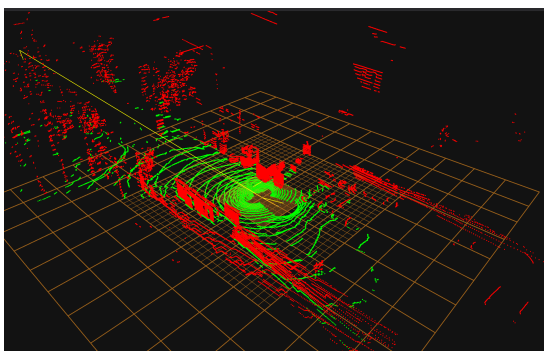
Рисунок 2 — Пример работы алгоритма разделения облака точек на точки земли и препятствий.
