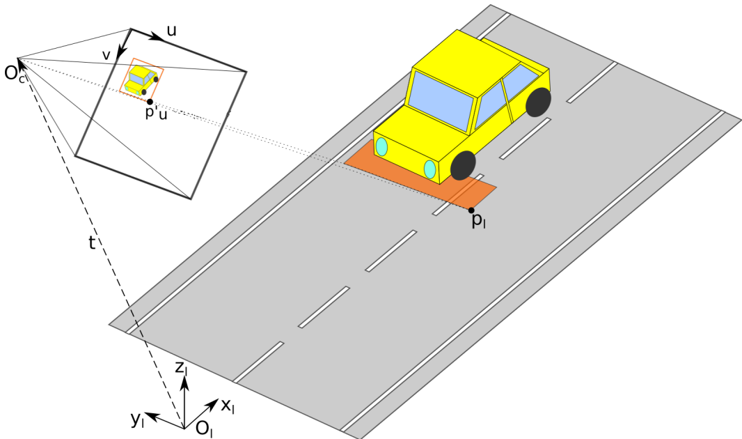
Рисунок 2.1 — Наивный подход к проецированию ограничивающей рамки в 2D на вид сверху.
