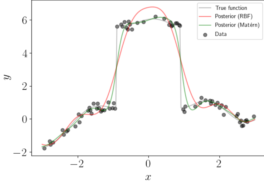
Рисунок 2.10 — Сравнение регрессии на основе гауссовских процессов с использованием в качестве ядра радиальной базисной функции и ядра Матерна [23]
