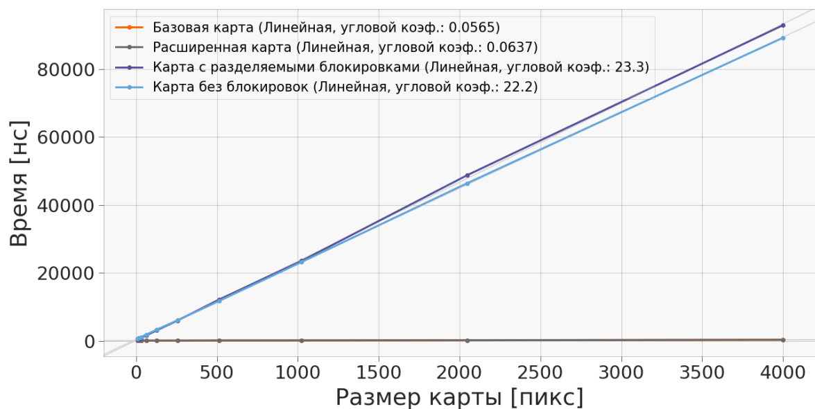
Рисунок 4.15 — График зависимости времени получения карты от её размера. График BaseOGM практически полностью совпадает с OMFWWithBuffer и на таком масштабе они не отличимы.
