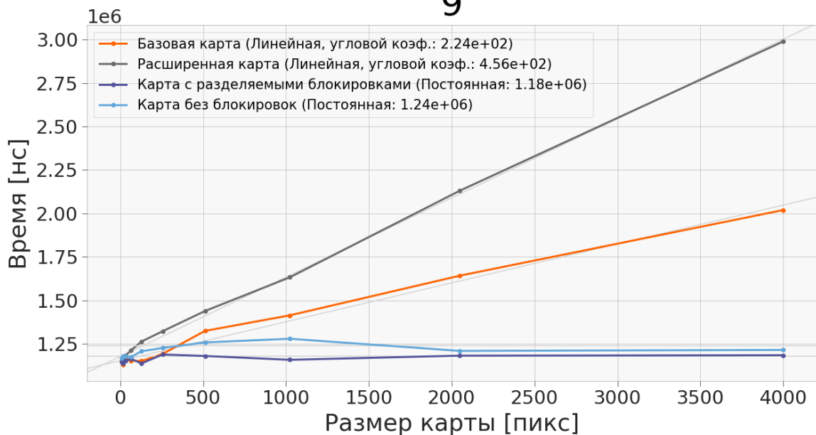
Рисунок 4.13 — График зависимости времени добавления фрагмента на карту в 9 потоках от размера карты.
