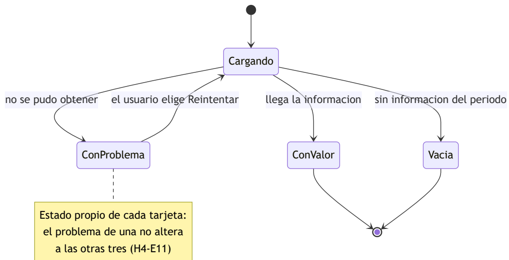
Diagrama (mermaid)
