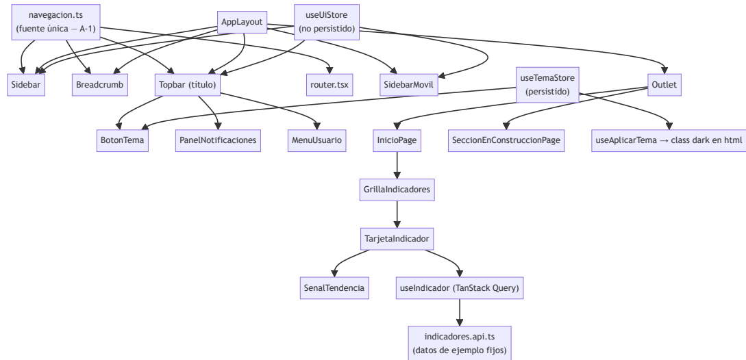
Diagrama (mermaid)
