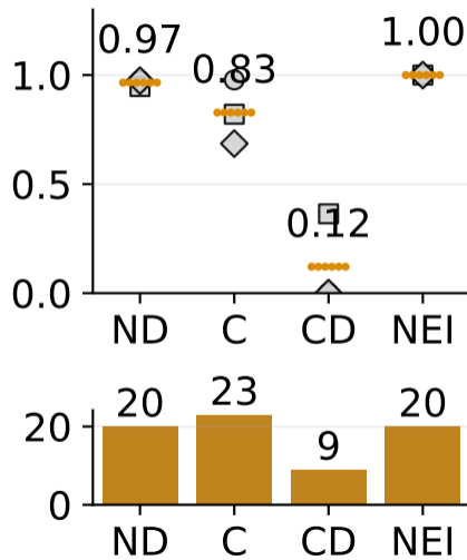
llama3.3:70b
