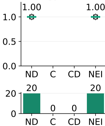
gpt-4o
