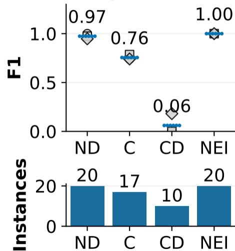
qwen:32b
