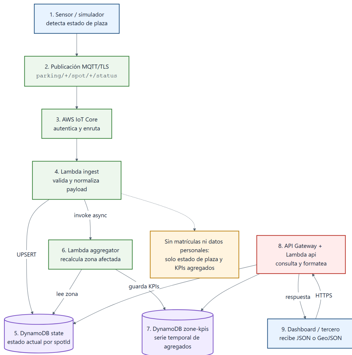
Figura 3: Flujo extremo a extremo desde el sensor hasta la API y el dashboard.
