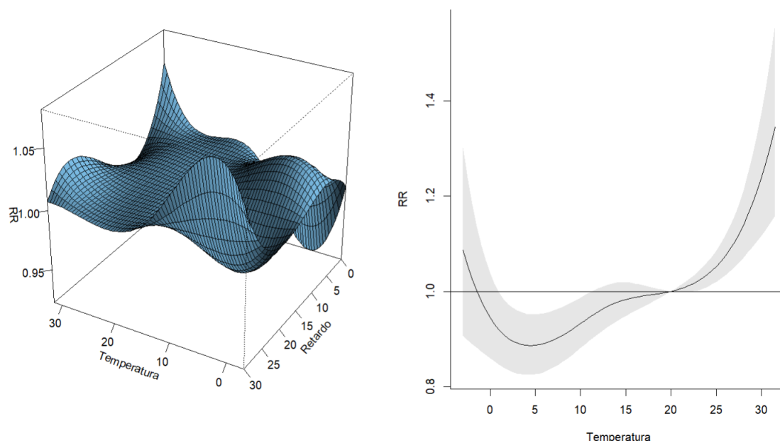
Figura 3.17: Gráficos correspondientes al modelo de Navarra cuya base utiliza B-splines con 4 grados de libertad para ambas dimensiones.
