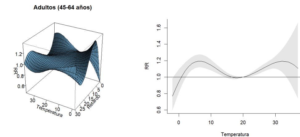
Figura A.3: Gráficos del análisis del grupo de 45-64 años.
