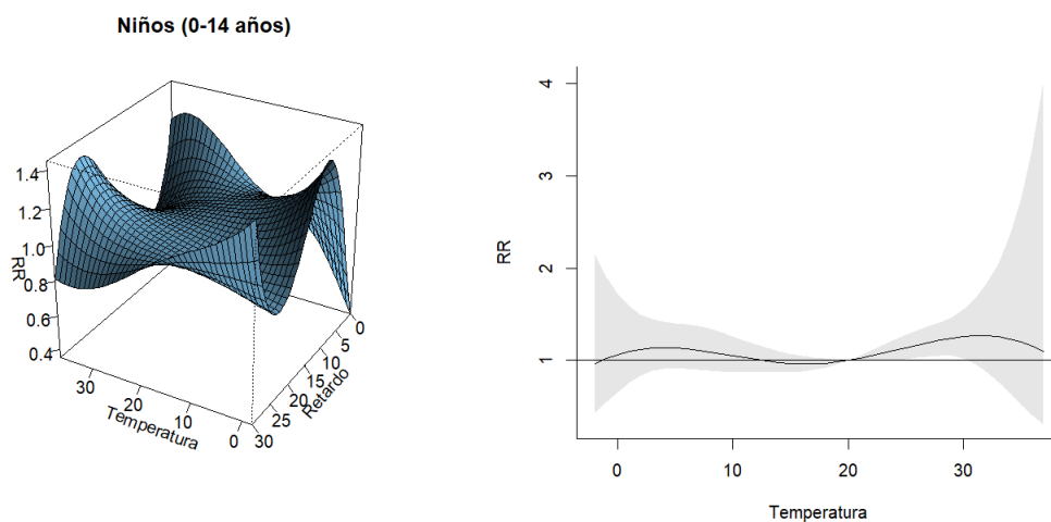
Figura A.1: Gráficos del análisis del grupo de 0-14 años.
