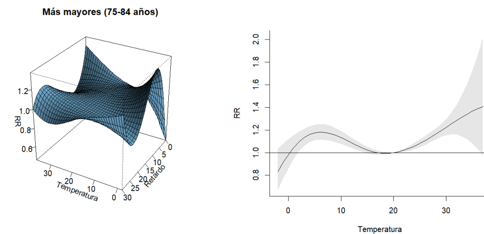
Figura A.5: Gráficos del análisis del grupo de 75-84 años.
