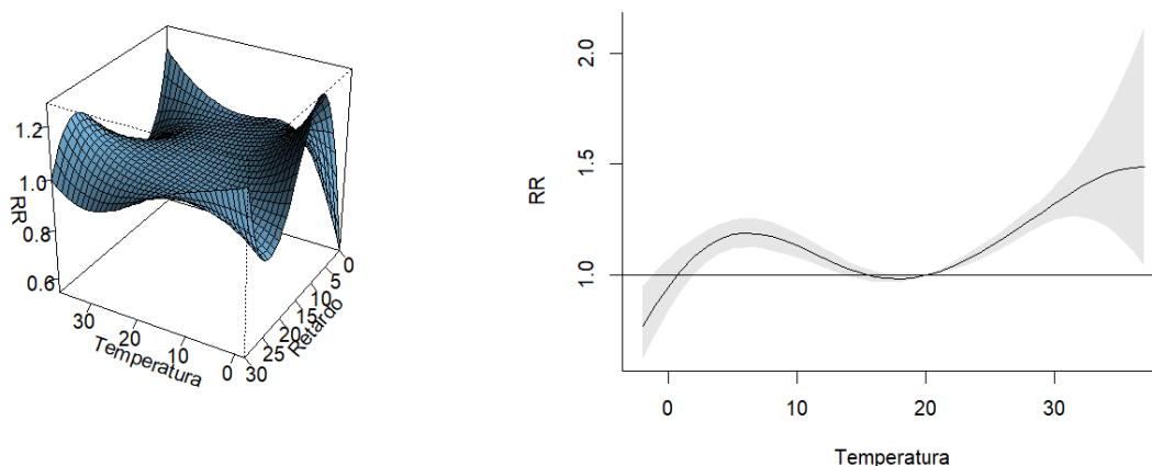
Figura 3.4: Gráficos correspondientes al grupo de población de más de 85 años de edad.
