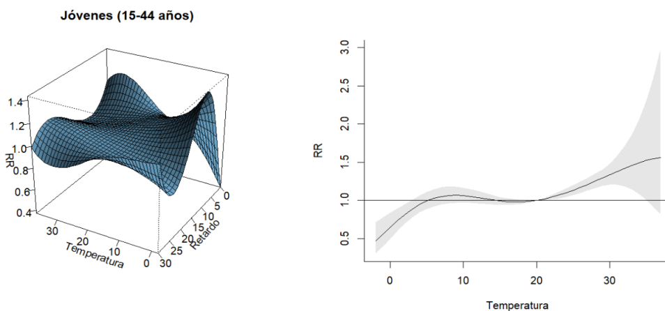
Figura A.2: Gráficos del análisis del grupo de 15-44 años.
