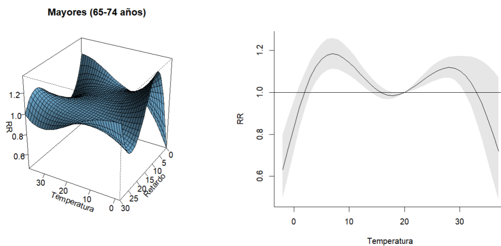
Figura A.4: Gráficos del análisis del grupo de 65-74 años.
