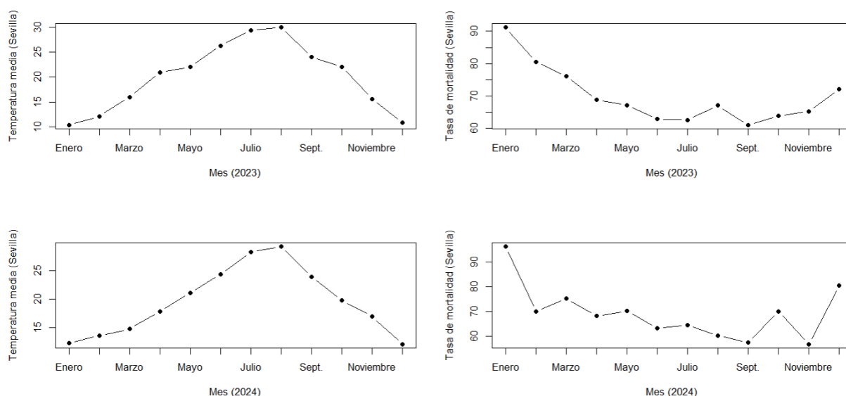
Figura 3.5: Gráficos que muestran las medias de las temperaturas medias y la tasa de mortalidad por 100000 habitantes por mes en 2023 y 2024 en Sevilla.
