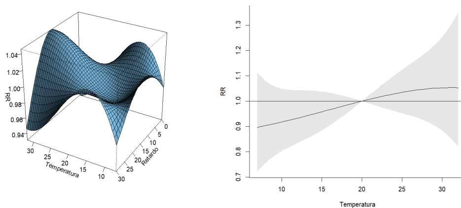
Figura 3.7: Gráficos del modelo que incluye un B-spline y un spline natural, ambos con 3 grados de libertad, para la temperatura y el retardo, respectivamente, con los datos de Sevilla del año 2024.
