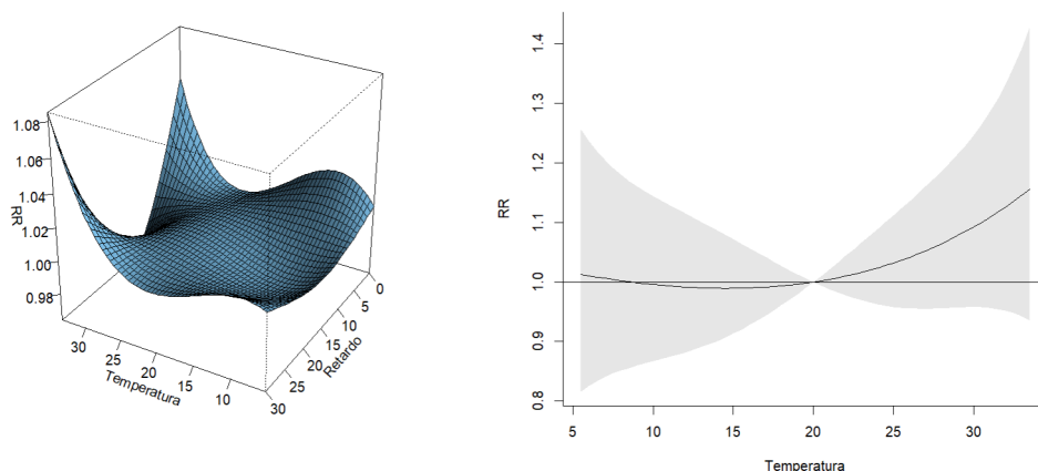
Figura 3.6: Gráficos del modelo que incluye un B-spline y un spline natural, ambos con 3 grados de libertad, para la temperatura y el retardo, respectivamente, con los datos de Sevilla del año 2023.
