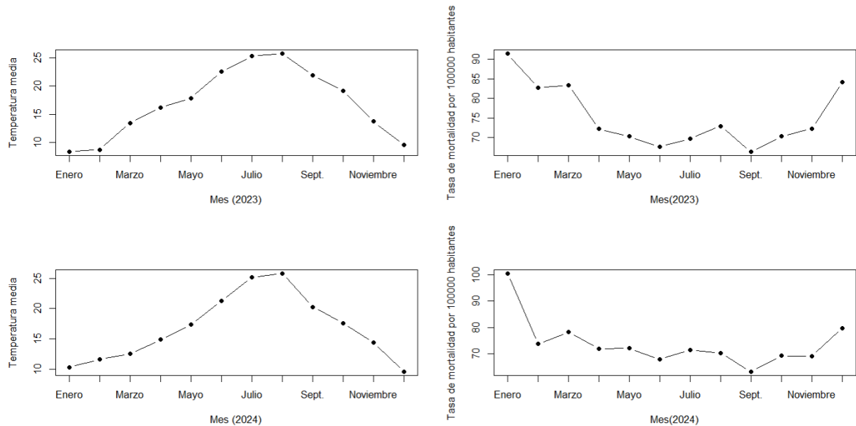
Figura 3.1: Gráficos que muestran las medias de las temperaturas medias (columna izquierda) y la tasa de mortalidad por 100000 habitantes (columna derecha) por mes en 2023 y 2024 en toda España.
