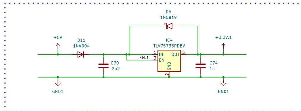
Regulador Lineal
