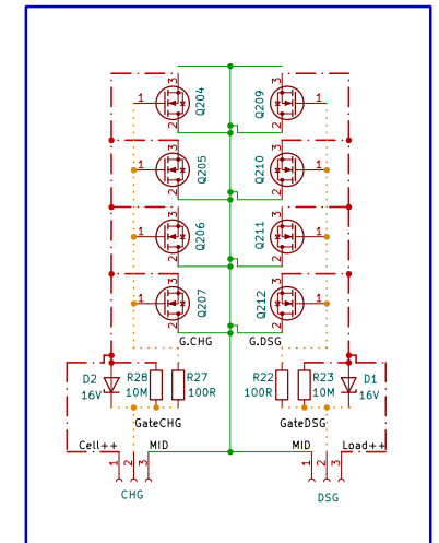
PCB_MOS
