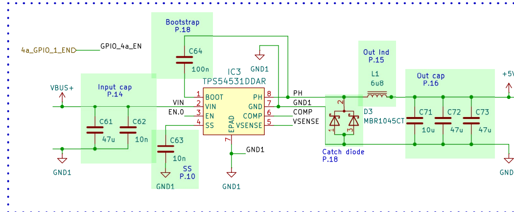
Convertidor Buck
