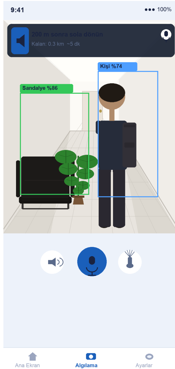
Şekil A.3. Algılama ekranı ve aktif navigasyon banner'ı
