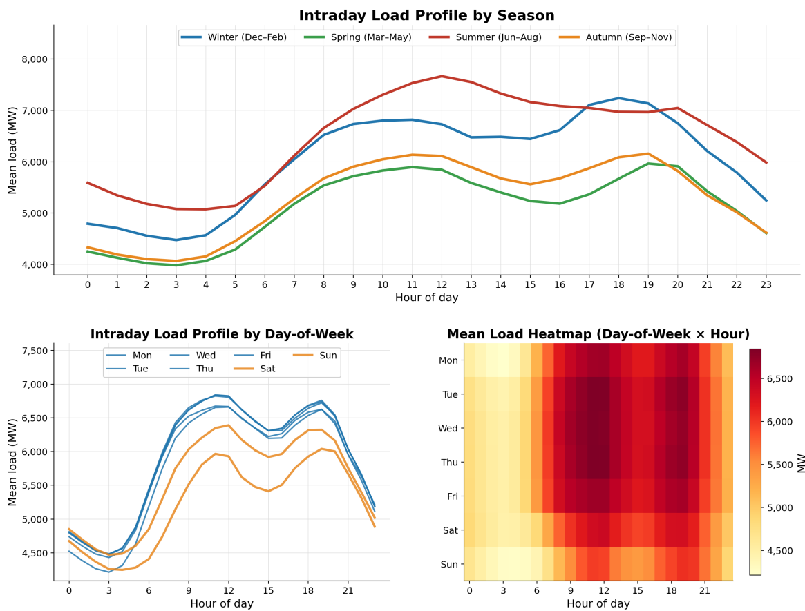
Σχήμα 3.6. Ενδοημερήσια μοτίβα ηλεκτρικού φορτίου, με ίδια διάταξη όπως η τιμή (Σχ. 3.5). Πάνω: προφίλ ανά εποχή· κάτω αριστερά: προφίλ ανά ημέρα εβδομάδας· κάτω δεξιά: θερμικός χάρτης μέσου φορτίου (ημέρα εβδομάδας \times ώρα).
