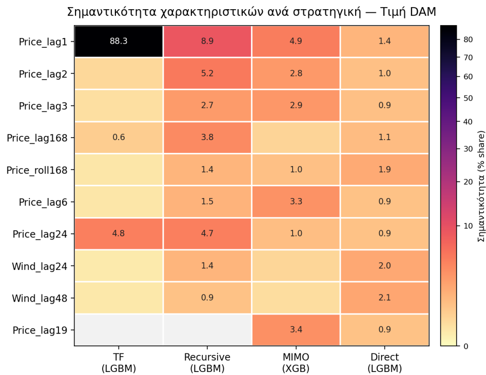
Σχήμα 7.9. Σημαντικότητα δέκα κορυφαίων χαρακτηριστικών ανά στρατηγική (πρωταθλητές gain), τιμή DAM. Ενιαία κλίμακα \text{PowerNorm}(\gamma = 0,45) , ώστε να φαίνονται οι μικρές τιμές δίπλα στο κορυφαίο 88%.
