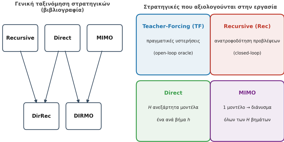
Σχήμα 2.5. Στρατηγικές πολυβηματικής πρόβλεψης. Αριστερά: η γενική ταξινόμηση της βιβλιογραφίας [28], με τις βασικές στρατηγικές (Recursive, Direct, MIMO) και τις υβριδικές παραλλαγές (DirRec, DIRMO). Δεξιά: οι τέσσερις στρατηγικές που αξιολογούνται στην παρούσα εργασία: Teacher-Forcing (TF) , Recursive (Rec) , Direct και MIMO .
