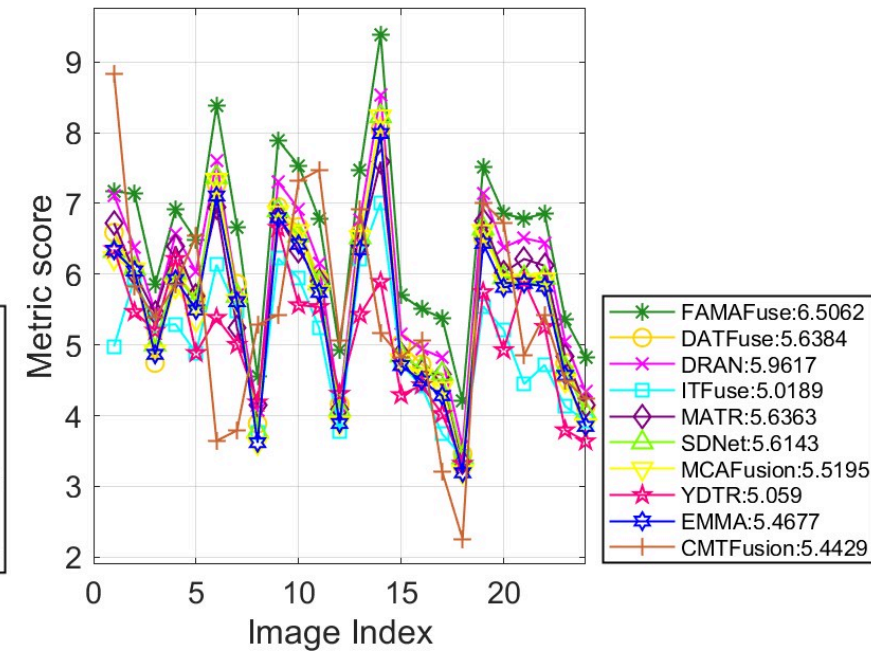
PSNR
