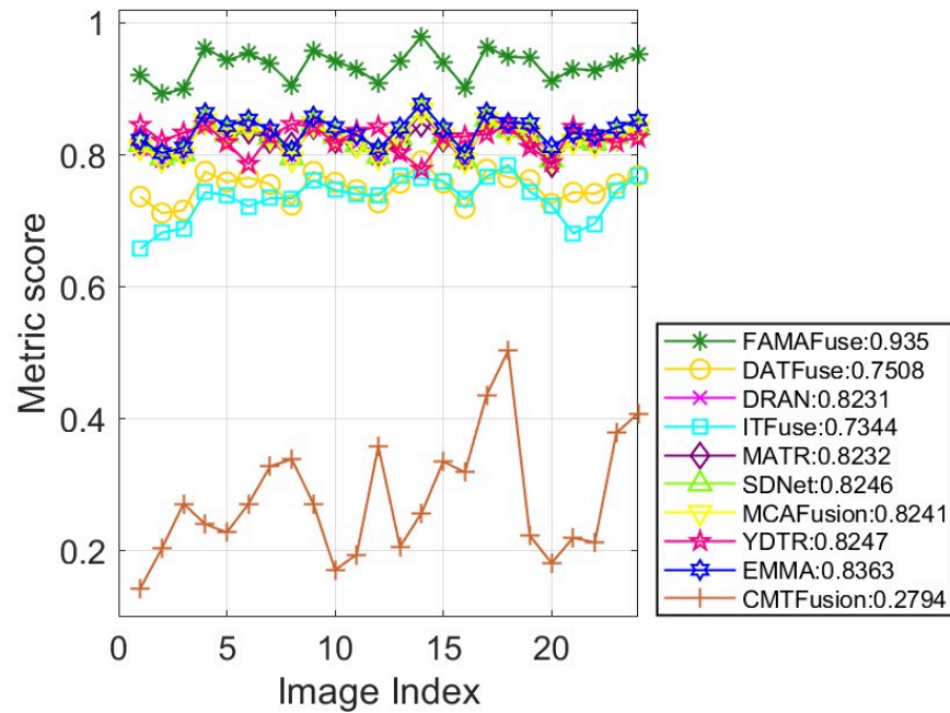
SSIM
