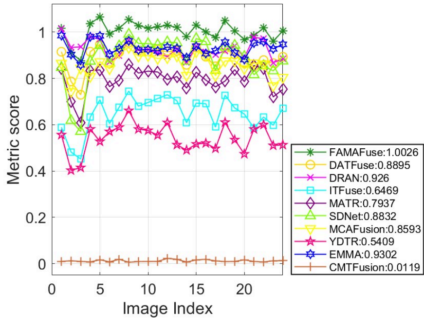
VIF
