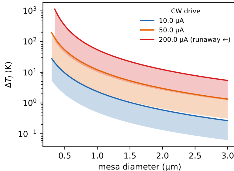
GaAs: T_J - T_{hs} @ 77 K (band: epi-k range)
