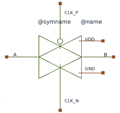
(b) Reusable Xschem symbol.
