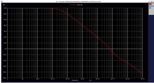
(a) Magnitudo gain diferensial.
