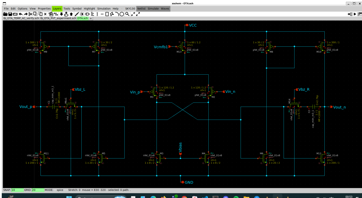
Figure 1: Skematik OTA baseline awal di Xschem sebelum penyederhanaan kompensasi direct-C. Cabang yang dikendalikan V_{bz} dan setting kapasitor kompensasi awal yang besar dipertahankan sebagai bagian dari riwayat desain.
