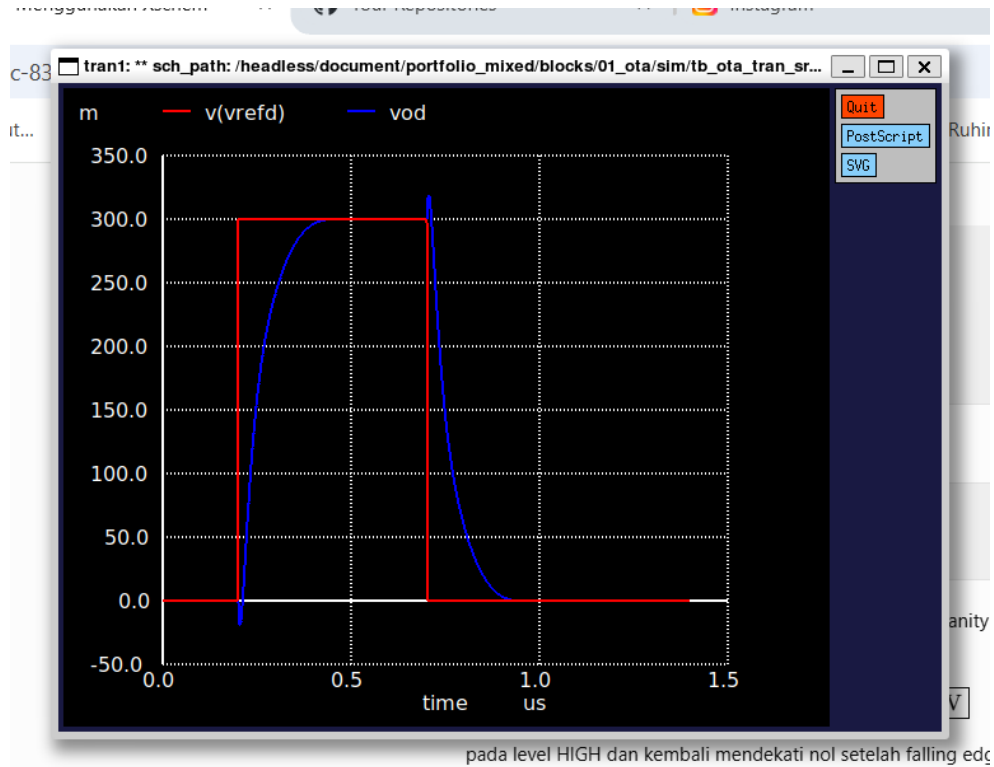
Figure 4: Respons diferensial large-signal untuk karakterisasi slew rate.
