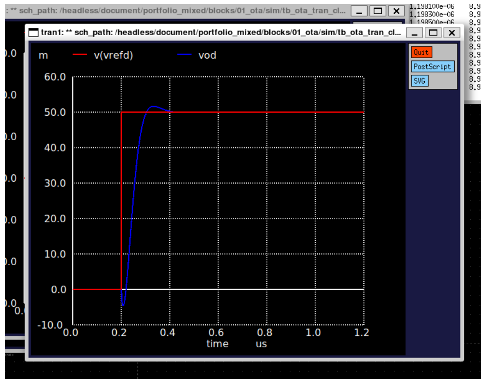
Figure 3: Respons closed-loop untuk step diferensial 50 mV.
