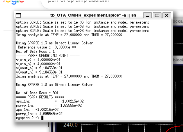
(b) Hasil PSRR+ nominal.
