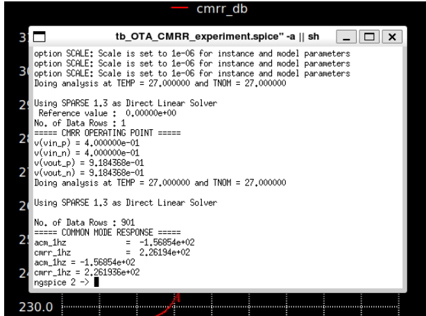
(a) Hasil CMRR nominal.
