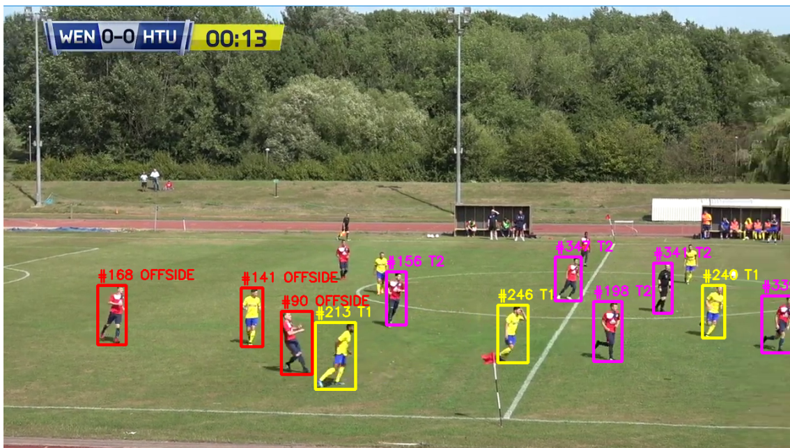
4.3. ábra. a 4.2 képen látható időpillanat a saját YOLO algoritmussal
