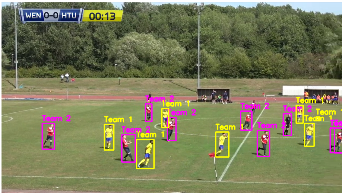
4.2. ábra. Egy képernyőkép a szoftver generikus YOLO-val történő futtatása során
