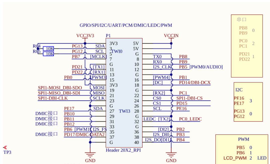
Рисунок 3 – Распиновка платы MangoPi MQ Pro
