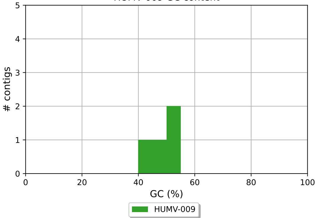
HUMV-009 GC content
