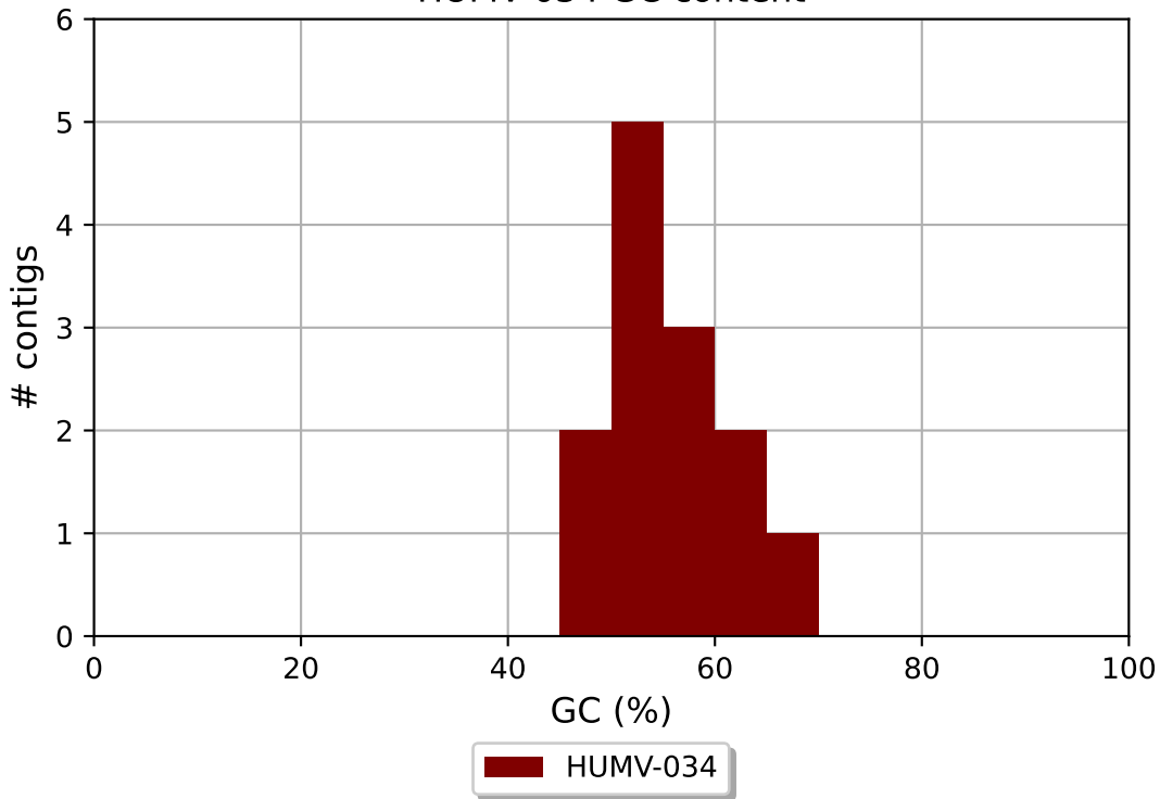
HUMV-034 GC content
