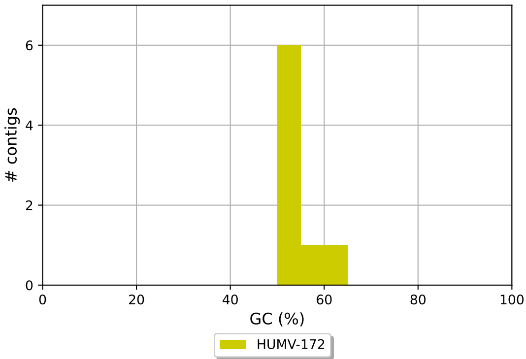
HUMV-172 GC content
