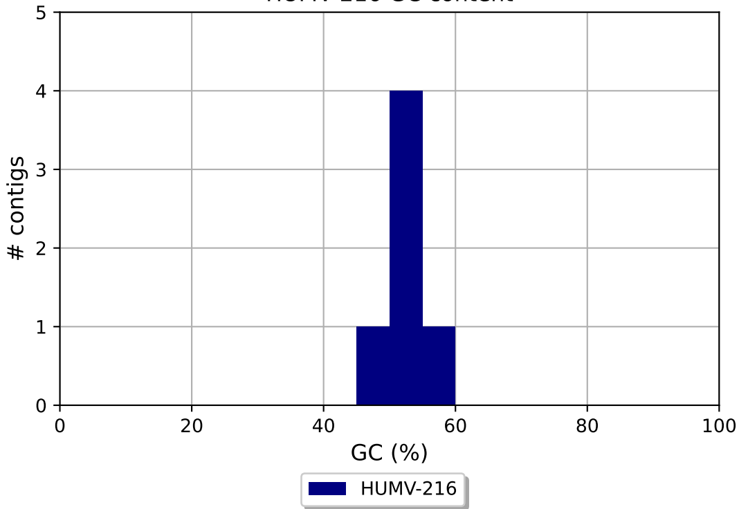
HUMV-216 GC content
