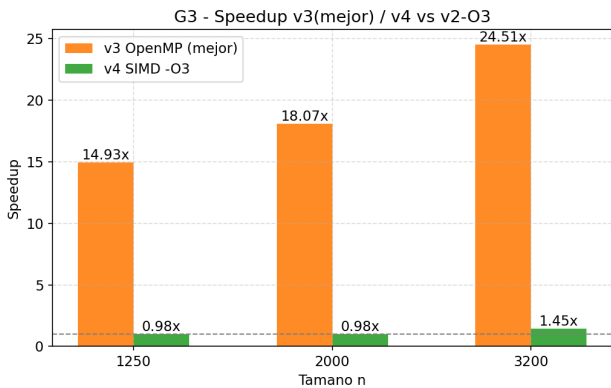
Figura 3: Speedup de la mejor configuración de v3 y de v4-03 respecto a v2-03.
