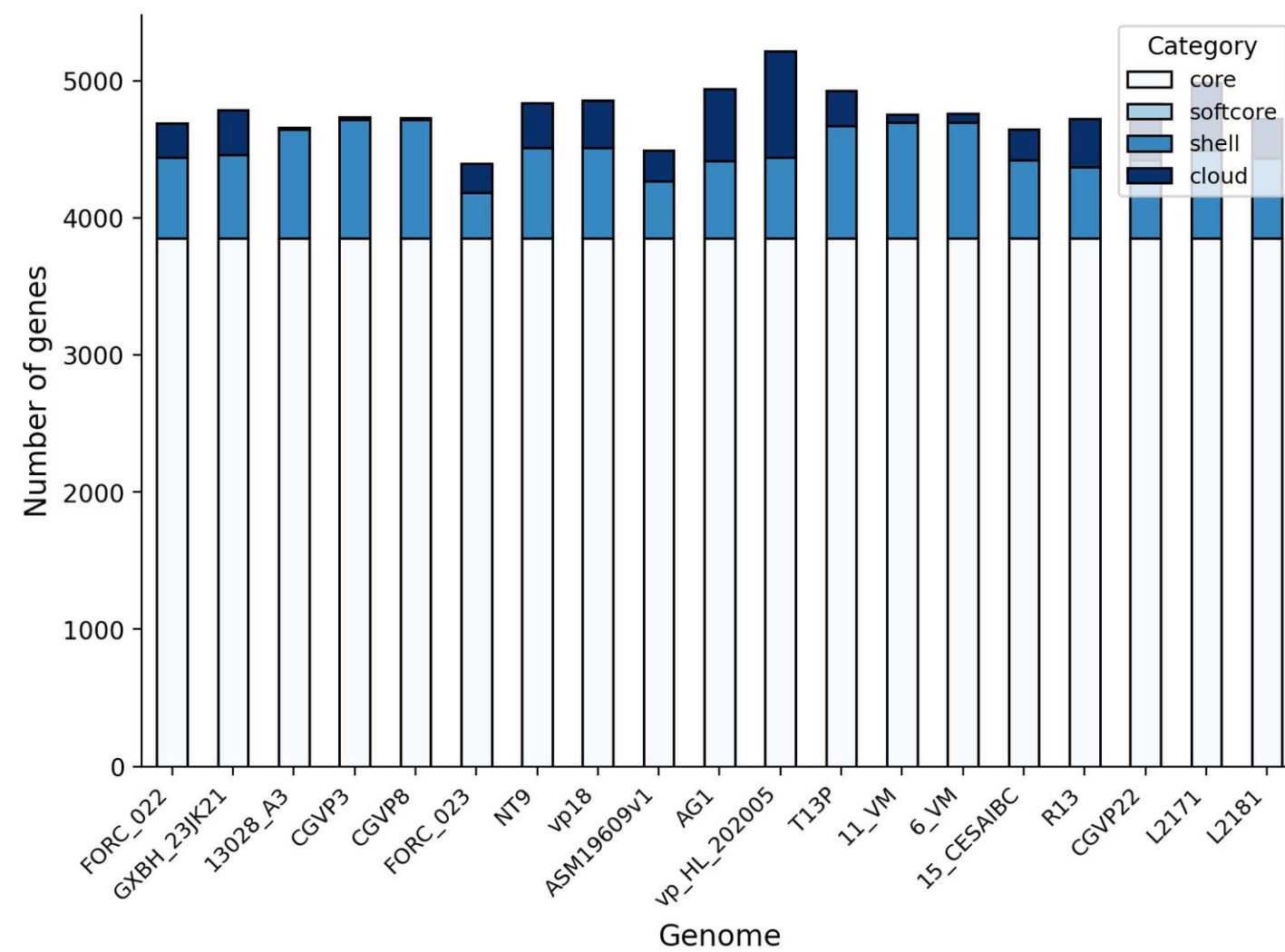
Gene categories per genome
