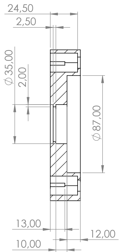
SECCIÓN A-A
