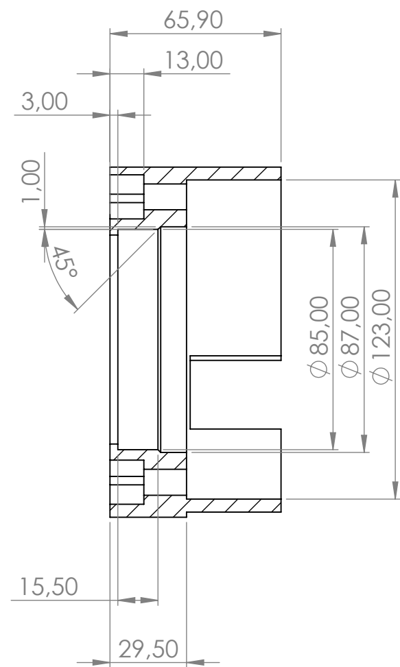
SECCIÓN A-A
