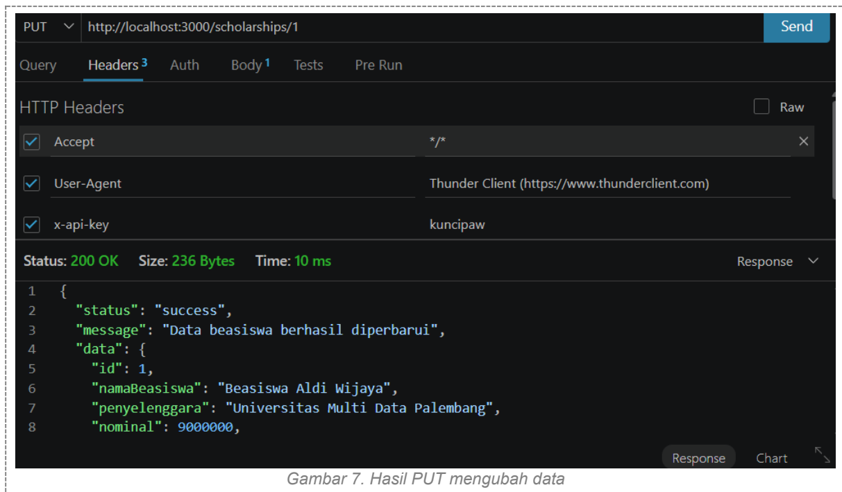
Gambar 7. Hasil PUT mengubah data
