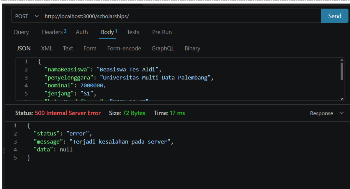
Gambar 11. POST dengan JSON rusak
