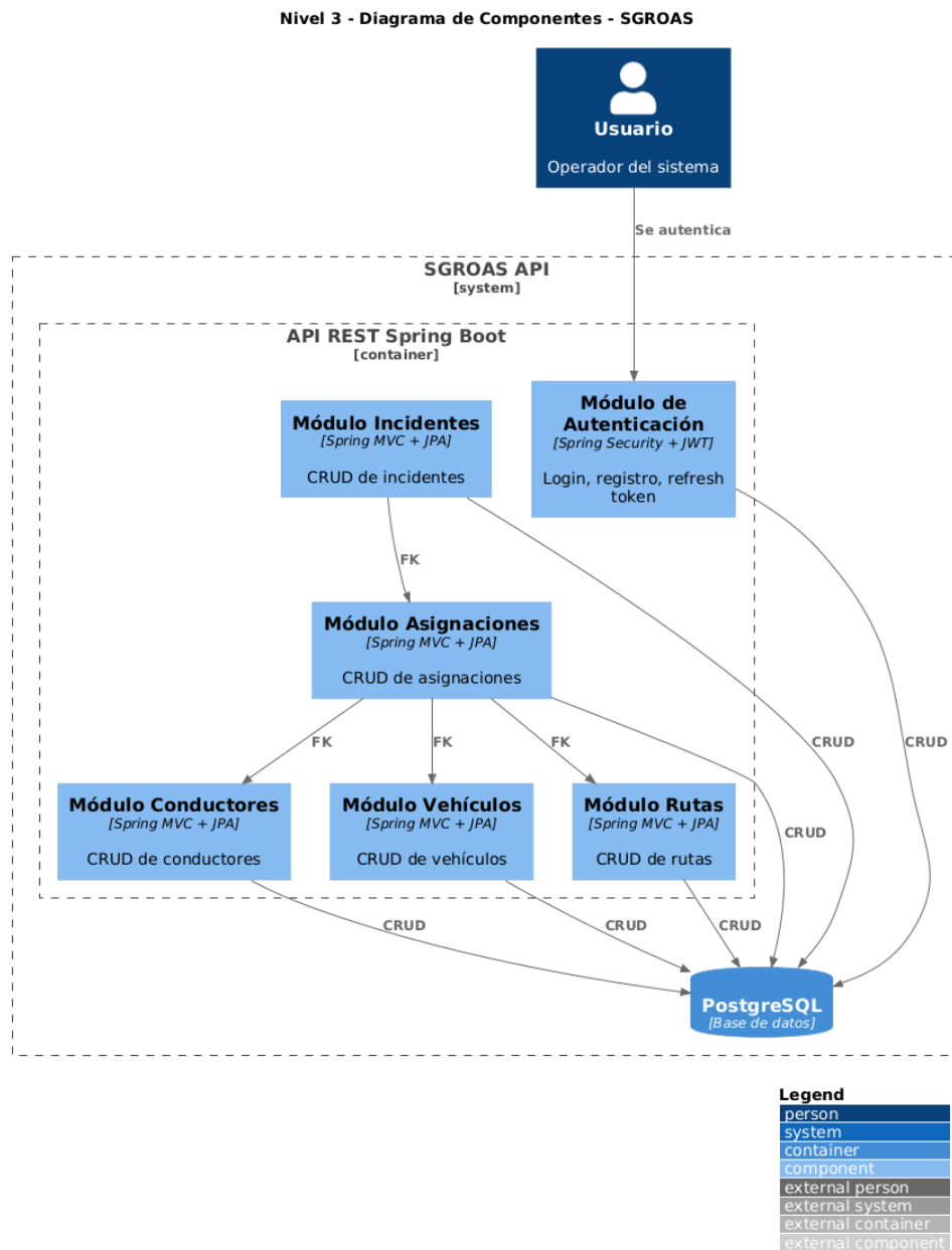
Figura 6.3: Diagrama C4 nivel 3 — Componentes del backend SGROAS.
