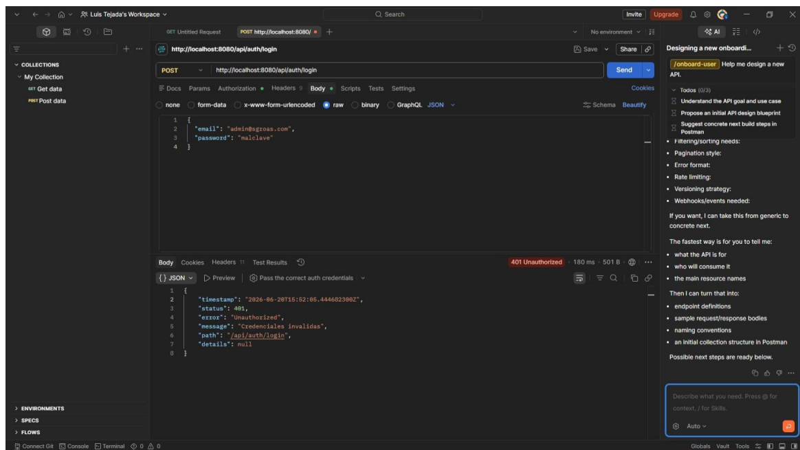
Figura 11. Acceso con credenciales invalidas.
